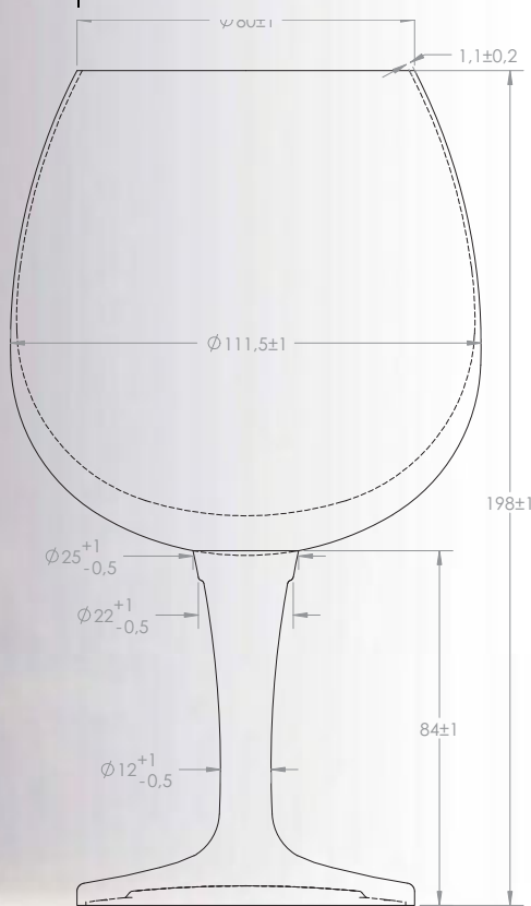
Technische Zeichnung Technical drawing
